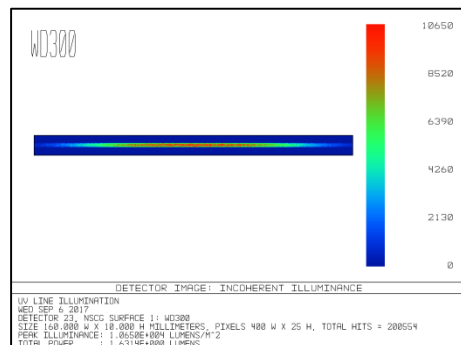
照度分布
